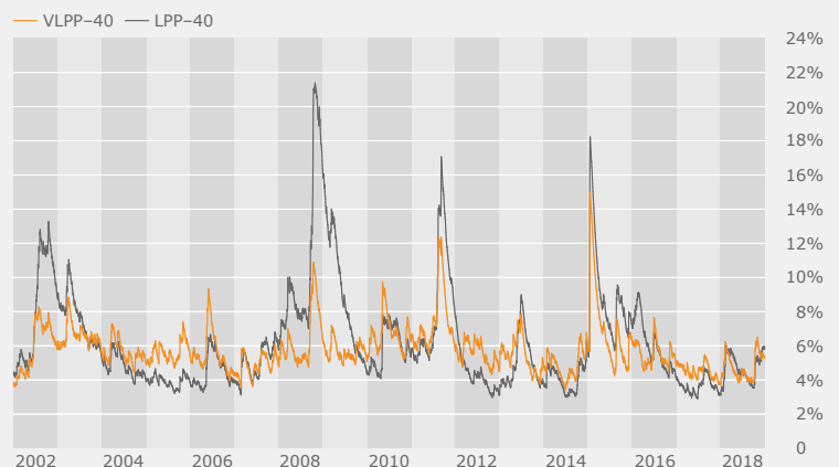
VLPP-40 vs LPP-40 Volatilité ex post 01.01.02-31.12.18
