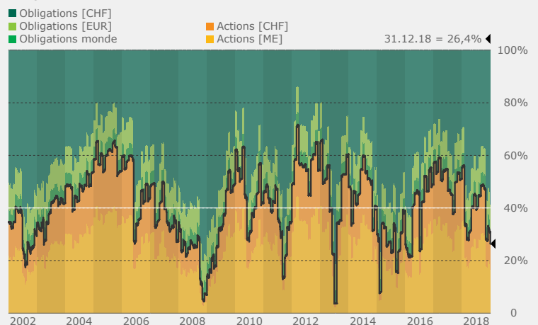
Fundo VLPP-40 Pondérations des classes d'actifs 01.01.02-31.12.18
