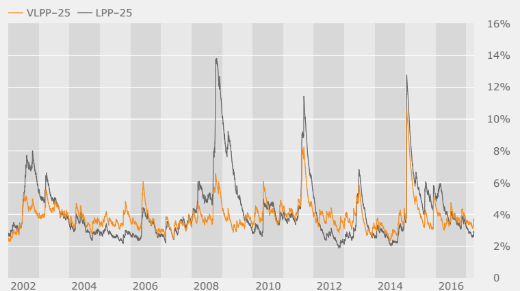
VLPP-25 vs LPP-25 Volatilité ex post 01.01.02–31.03.17
