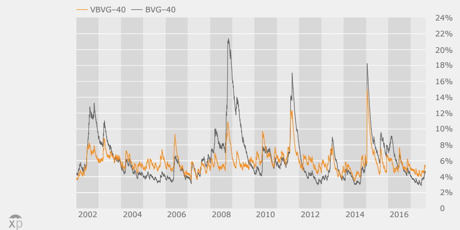
VBVG-40 vs BVG-40 Ex-post Volatilität 01.01.02–31.08.17
