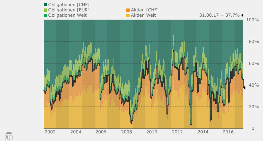
Fundo VBVG-40 Gewichtung Anlageklassen 01.01.02–31.08.17
