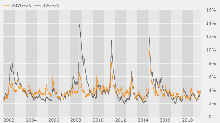
VBVG-25 vs BVG-25 Ex-post Volatilität 01.01.02–30.08.19
