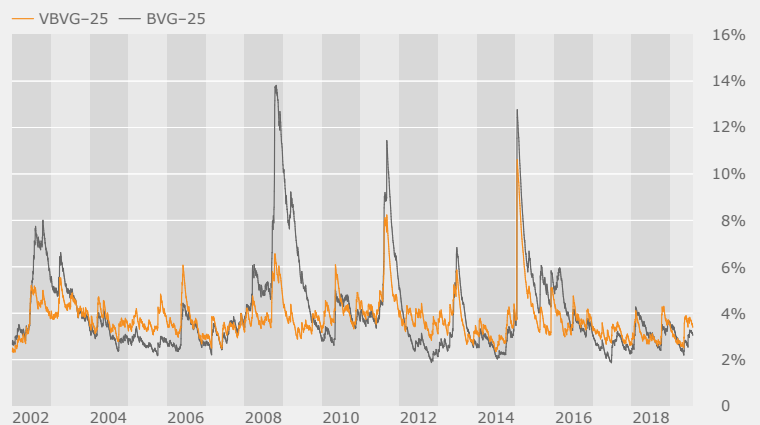
VBVG-25 vs BVG-25 Ex-post Volatilität 01.01.02–31.07.19
