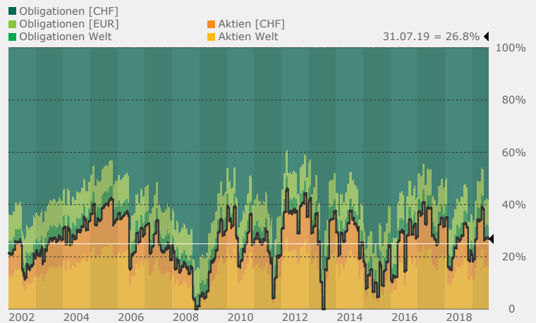
Fundo VBVG-25 Gewichtung Anlageklassen 01.01.02–31.07.19
