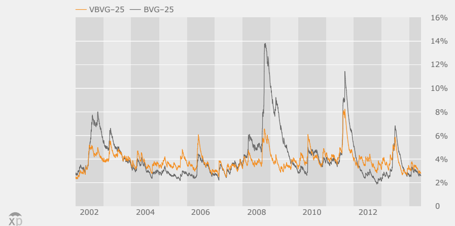
VBVG-25 vs BVG-25 Ex-post Volatilität 01.01.02–30.05.14
