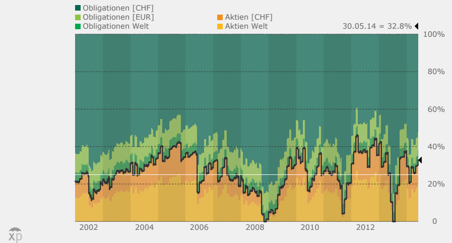
Fundo VBVG-25 Gewichtung Anlageklassen 01.01.02–30.05.14
