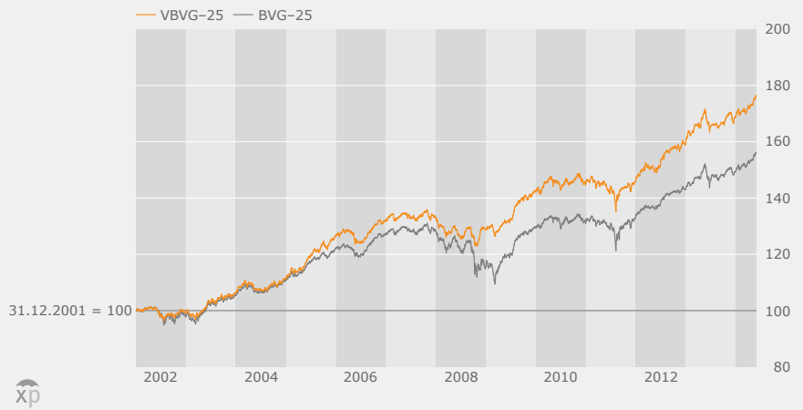
Fundo VBVG-25 vs BVG-25 01.01.02–30.05.14
