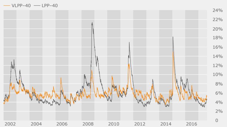
VLPP-40 vs LPP-40 Volatilité ex post 01.01.02–31.08.17
